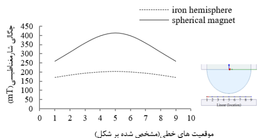
شکل ۱۰) توزیع چگالی شار مغناطیسی در فاصله ۲ میلی‌متر از سطح نیم کره به صورت خطی (شبیه سازی)
