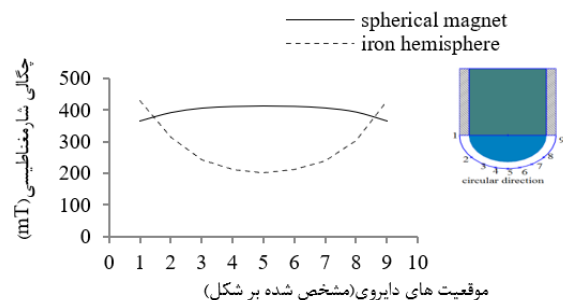
شکل ۱۱) توزیع چگالی شار مغناطیسی در فاصله ۲ میلی‌متر از سطح نیم کره به صورت دایره ای (شبیه سازی)
