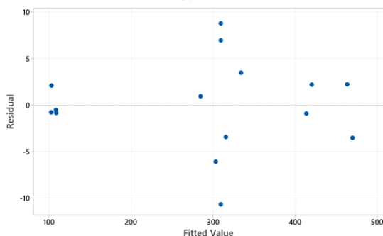
شکل ۱۵) پراکندگی باقیمانده‌های سایش جانبی نسبت به مدل منطبق شده
