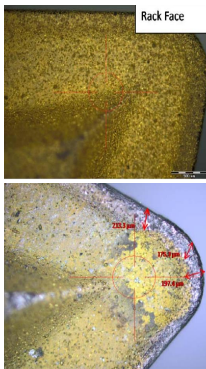
شکل ۱۱) ابزار قبل و بعد از عملیات تراشکاری
