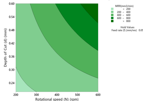
شکل ۸) نمودار برهم کنش سرعت دوران اسپیندل و عمق برشی بر روی رفتار نرخ براده برداری
