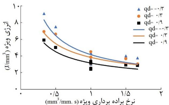
شکل ۴) نمودار تغییرات انرژی مخصوص سنگ‌زنی با تغییر در نرخ براده برداری ویژه GFRP
