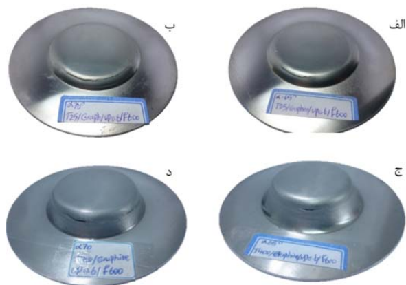
شکل ۲۱) نمونه‌های شکل‌داده شده با گام عمودی ۰/۶ میلی‌متر و سرعت پیش‌روی ۶۰۰ میلی‌متر بر دقیقه در، الف) دمای ۲۵ درجه سانتی‌گراد و زاویه دیواره ۶۰ درجه، ب) دمای ۲۵ درجه سانتی‌گراد و زاویه دیواره ۷۰ درجه، ج) ۴۰۰ درجه سانتی‌گراد و زاویه دیواره ۶۰ درجه، د) ۴۰۰ درجه سانتی‌گراد و زاویه دیواره ۷۰ درجه
