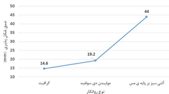
نمودار ۴) منحنی تاثیر نوع روانکار بر عمق شکل‌پذیری در زاویه ۶۰ درجه، دمای ۴۰۰ درجه سانتی‌گراد، گام عمودی ۶/۰ میلی‌متر، سرعت پیش‌روی ۱۰۰ میلی‌متر بر دقیقه در حالت‌های مختلف روانکاری
