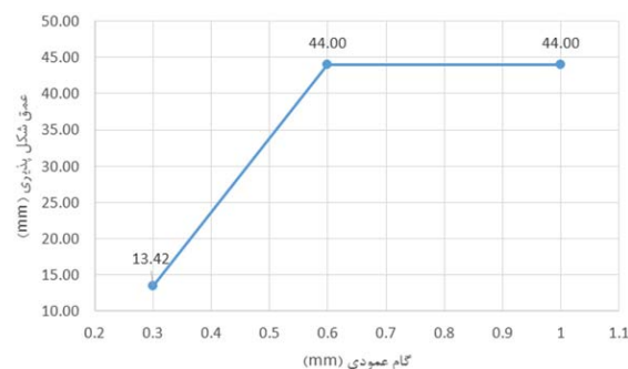
نمودار ۵) نمودار تاثیر گام عمودی بر عمق شکل‌پذیری در زاویه ۶۰ درجه، دمای ۴۰۰ درجه سانتی‌گراد، سرعت پیش‌روی ۱۰۰ میلی‌متر بر دقیقه با استفاده از روانکار پودر گرافیت در گام‌های عمودی مختلف
