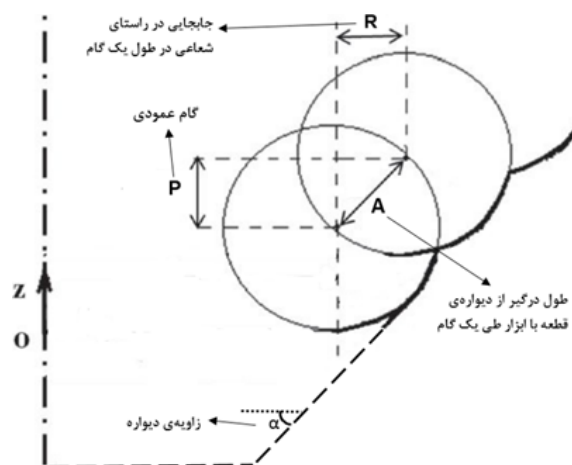
شکل ۱۹) نحوه حرکت ابزار در یک گام کامل [22]
