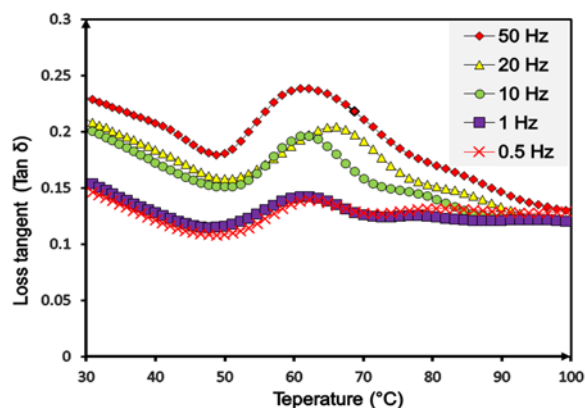
نمودار ۵) تانژانت اتلاف ماده TPU در بسامدهای ۵۰، ۲۰، ۱۰، ۱، ۰/۵ و ۰/۱ هرتز و آهنگ تغییرات دما ۲ درجه سانتی‌گراد بر دقیقه
