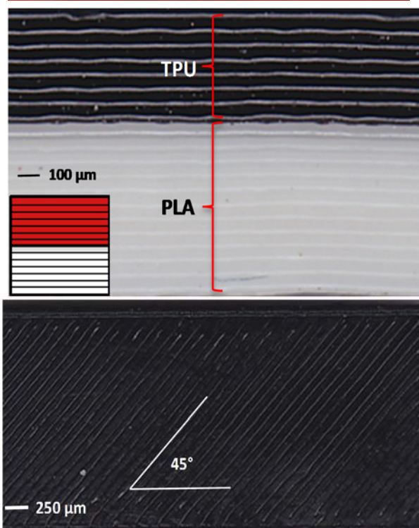
شکل ۳) از بالا به پایین به‌ترتیب نمونه چاپ‌شده با ابعاد ۶×۱۰×۵۰ میلی‌متر، نمای جانبی و نحوه اتصال لایه‌های PLA و TPU به یکدیگر، راستای پرینت با زاویه ۴۵ درجه
