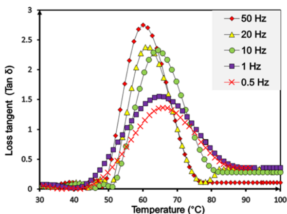
نمودار ۱) تانژانت اتلاف ماده PLA در بسامدهای ۵/۵، ۱۰، ۲۰ و ۵۰ هرتز و آهنگ تغییرات دما ۲ درجه سانتی‌گراد بر دقیقه
