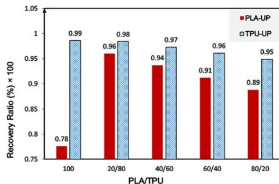
نمودار ۷) نسبت بازیابی در سیکل‌های ترمومکانیکی برای نسبت‌های وزنی مختلف و لایه‌چینی‌های TPU-UP و PLA-UP
