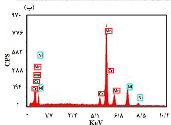
شکل ۴ (الف) تصویر میکروسکوپ الکترونی روبشی از نمونه تغییرشکل یافته در دمای ۹۰۰ درجه سانتی‌گراد و سرعت کرنش ۰/۱ بر ثانیه و (ب) آنالیز طیف‌سنجی انرژی پرتو ایکس از نقطه نشان داده شده روی ذره فاز دوم در شکل (الف)
