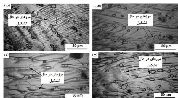
شکل ۶) تصاویر ریزساختاری نمونه‌ها پس از آزمون فشار گرم در دمای ۹۵۰ و تحت نرخ کرنش‌های: (الف) ۰/۰۰۱ \text{ s}^{-1} ، (ب) ۰/۰۱ \text{ s}^{-1} ، (ج) ۰/۱ \text{ s}^{-1} و (د) ۱ \text{ s}^{-1} .
