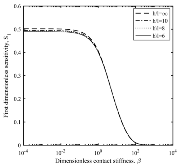
نمودار (۳) اولین حساسیت خمشی در برابر سختی تماسی
