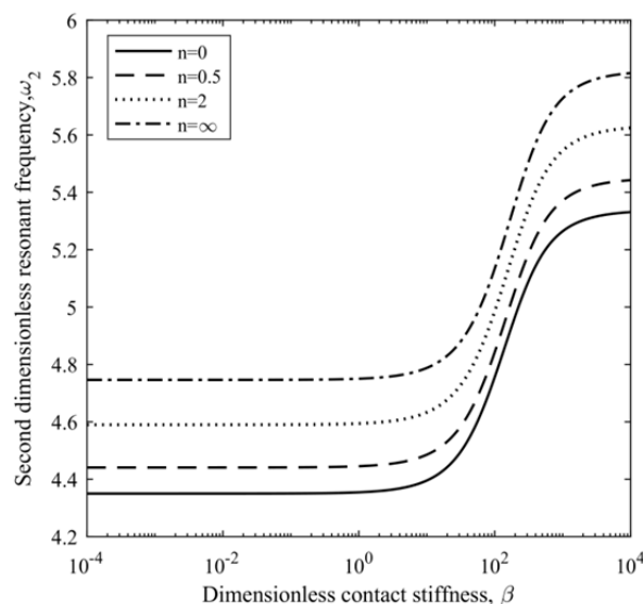
نمودار ۶) دومین فرکانس تشدید از میکروتیر مواد مندرج تابعی
