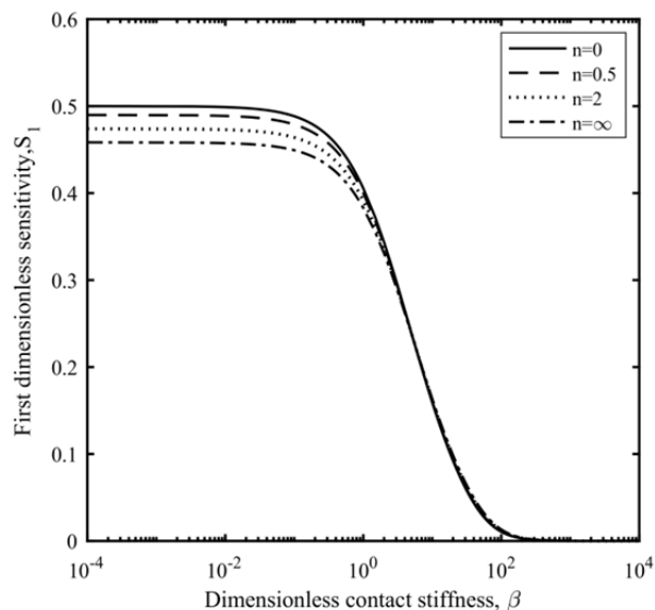
نمودار ۷) اولین حساسیت خمشی از میکروتیر مواد مندرج تابعی
