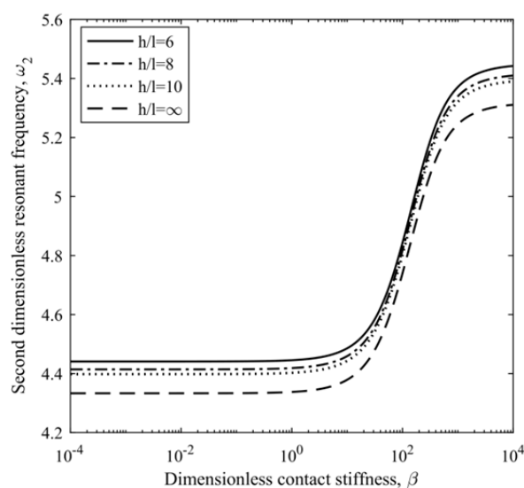
نمودار (۲) دومین فرکانس تشدید در برابر سختی تماسی
