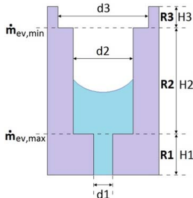
شکل ۲) طرحواره میکروکانال پیشنهادی با سطح مقطع غیریکنواخت
