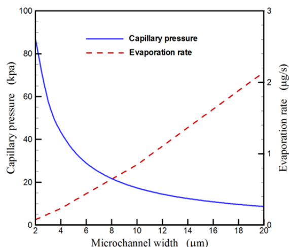
نمودار ۵) مقادیر فشار مویینگی و بیشینه نرخ تبخیر در بخش تبخیرکننده برحسب عرض میکروکانال
