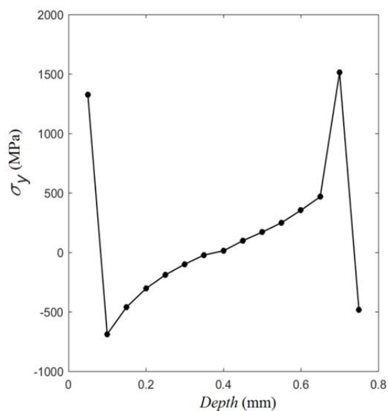
نمودار ۱۲) توزیع تنش پسماند غیریکنواخت \sigma_y در برآزش منحنی درجه دو
