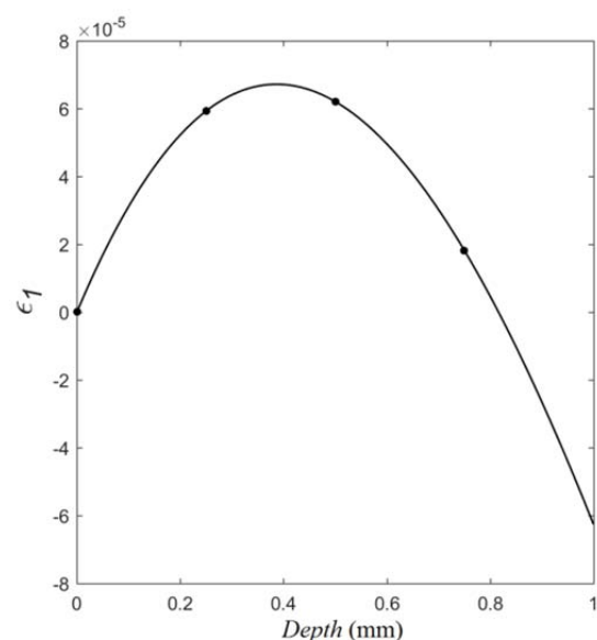
نمودار ۱۵) برازش منحنی درجه سه به کرنش \varepsilon_1 در راستای صفر درجه
