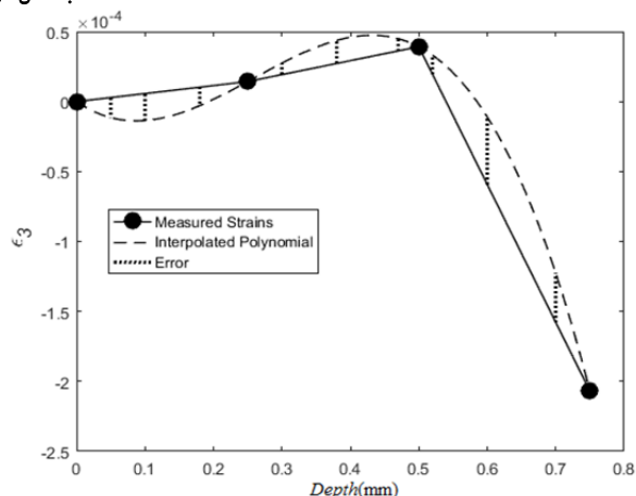
نمودار ۲۳) شماتیک خطی ناشی از برازش منحنی درجه سه برای کرنش ( \epsilon_z )
