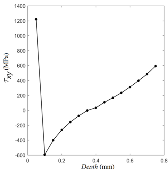
نمودار ۱۳) توزیع تنش پسماند غیریکنواخت \tau_{xy} در برآزش منحنی درجه دو
