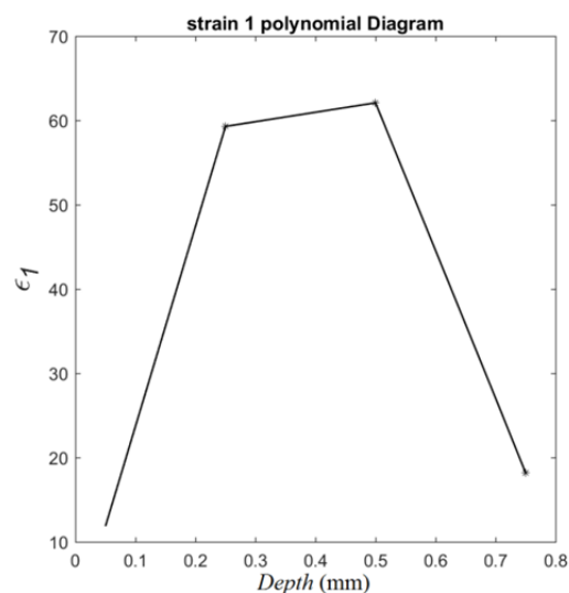
نمودار ۱) برآزش خطی کرنش \epsilon_1 در راستای صفدرجه
