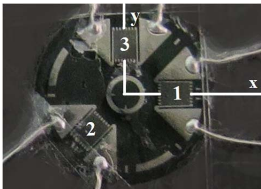
شکل ۱) شماتیک از یک کرنش‌سنج روزت
