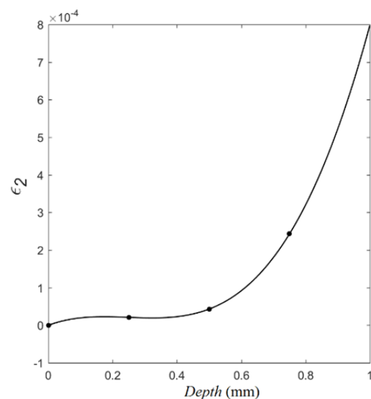
نمودار ۱۶) برازش منحنی درجه سه به کرنش \varepsilon_2 در راستای ۴۵ درجه
