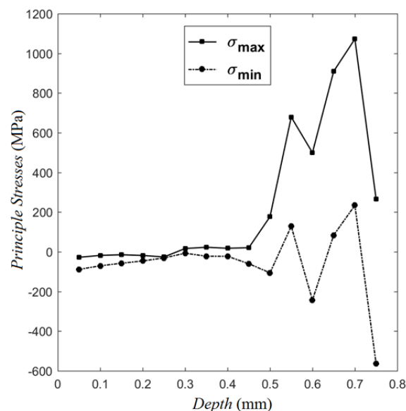
نمودار ۷) تنش‌های اصلی در برازش خطی
