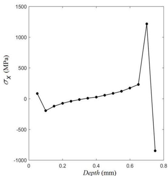
نمودار ۱۱) توزیع تنش پسماند غیریکنواخت \sigma_x در برآزش منحنی درجه دو
