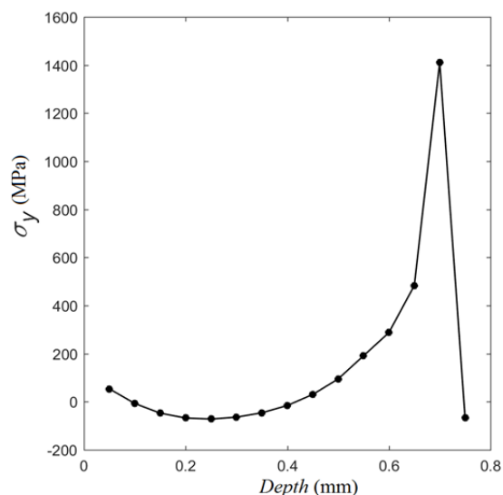
نمودار ۱۹) توزیع تنش پسماند غیریکنواخت \sigma_y در برآزش منحنی درجه سه
