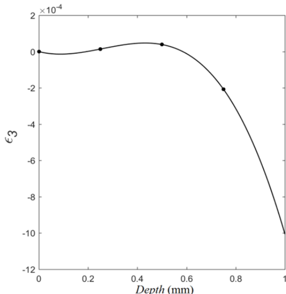
نمودار ۱۷) برازش منحنی درجه سه به کرنش \varepsilon_3 در راستای ۹۰ درجه
