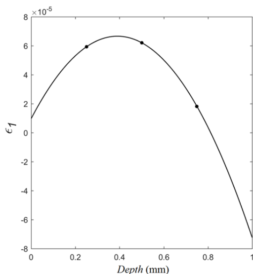
نمودار ۸) برازش منحنی درجه دو به کرنش \epsilon_1 در راستای صف درجه
