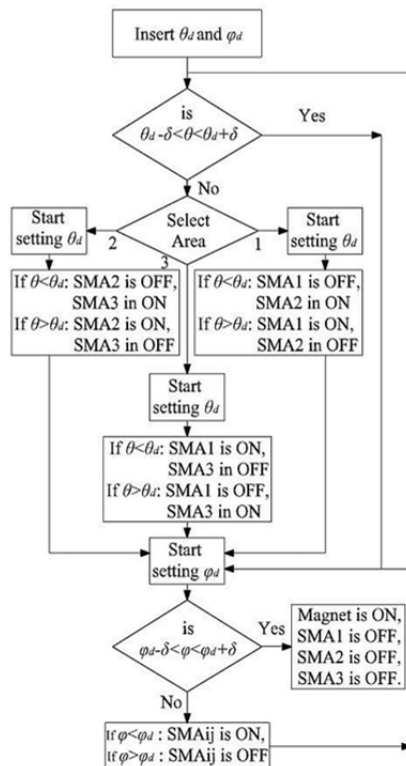
شکل ۱۰) الگوریتم کنترل موقعیت مازول با سیستم تثبیت موقعیت
