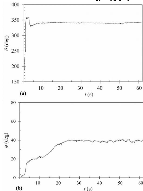
نمودار ۷ موقعیت‌دهی مازول برای زاویه \theta_d = 340^\circ و \phi_d = 40^\circ بدون استفاده از سیستم تثبیت‌کننده موقعیت؛ (a) \theta_d = 340^\circ , (b) \phi_d = 40^\circ
