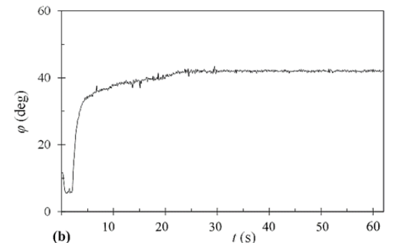
نمودار ۱۰) موقعیت‌دهی مازول برای زاویه \theta_d = 340^\circ و \phi_d = 40^\circ با استفاده از سیستم تثبیت‌کننده موقعیت: (a) \theta_d = 340^\circ , (b) \phi_d = 40^\circ
