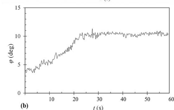
نمودار ۳) موقعیت‌دهی ماژول برای زاویه \theta_d=200^\circ و \varphi_d=30^\circ با کاربرد یک محرک فنری در هر جهت: (a) \theta_d=200^\circ , (b) \varphi_d=30^\circ
