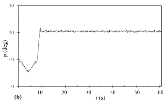
نمودار ۹) موقعیت‌دهی مازول برای زاویه \theta_d = 60^\circ و \phi_d = 20^\circ با استفاده از سیستم تثبیت‌کننده موقعیت: (a) \theta_d = 60^\circ , (b) \phi_d = 20^\circ
