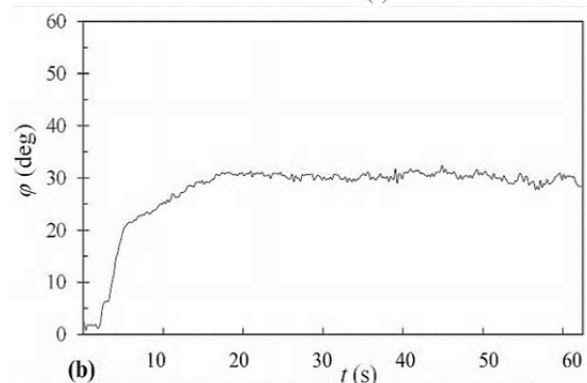
نمودار ۵) موقعیت‌دهی ماژول برای زاویه \theta_d=200^\circ و \varphi_d=30^\circ بدون استفاده از سیستم تثبیت‌کننده موقعیت: (a) \theta_d=200^\circ , (b) \varphi_d=30^\circ
