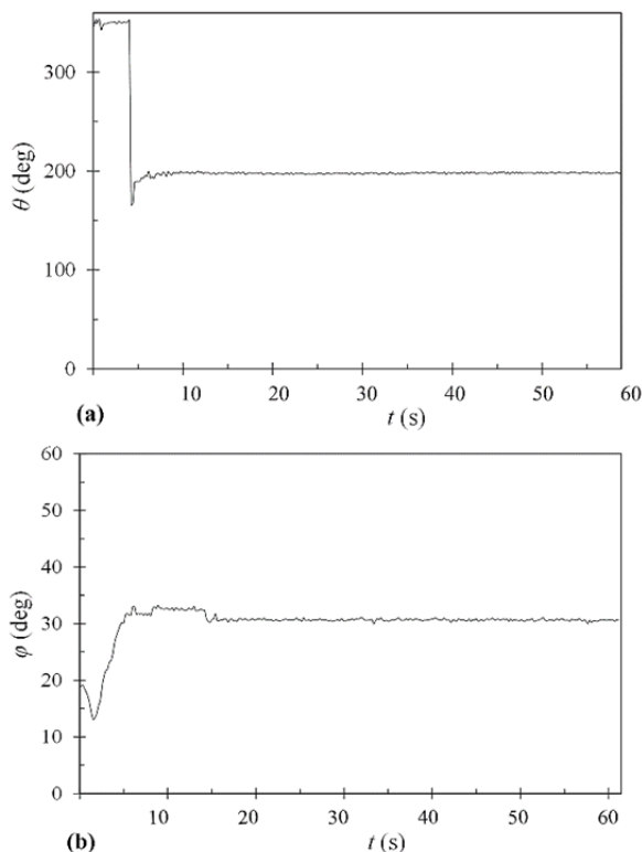
نمودار ۸ موقعیت‌دهی مازول برای زاویه \theta = 200^\circ و \phi = 30^\circ با استفاده از سیستم تثبیت‌کننده موقعیت؛ (a) \theta_d = 200^\circ , (b) \phi_d = 30^\circ
