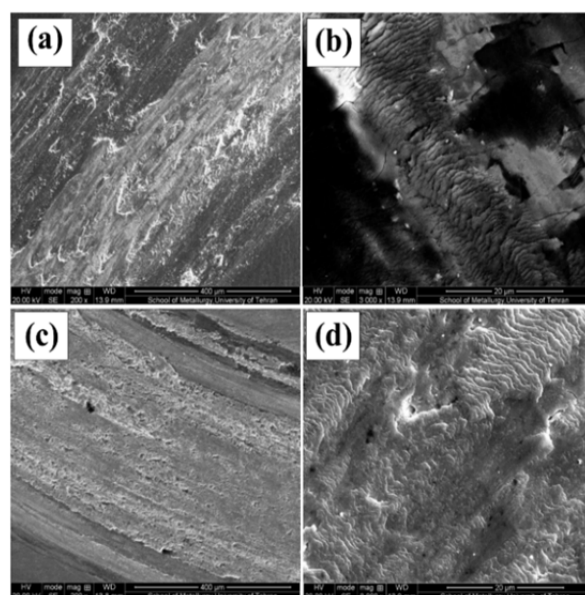
شکل ۶) تصویر SEM سطح سایش قبل از عملیات حرارتی با پوشش گرادانی نیکل - فسفر و پوشش گرادانی نیکل - فسفر - آلومینا؛ (a, b) قبل از عملیات حرارتی با پوشش گرادانی نیکل - فسفر، (c, d) پوشش گرادانی نیکل - فسفر - آلومینا
