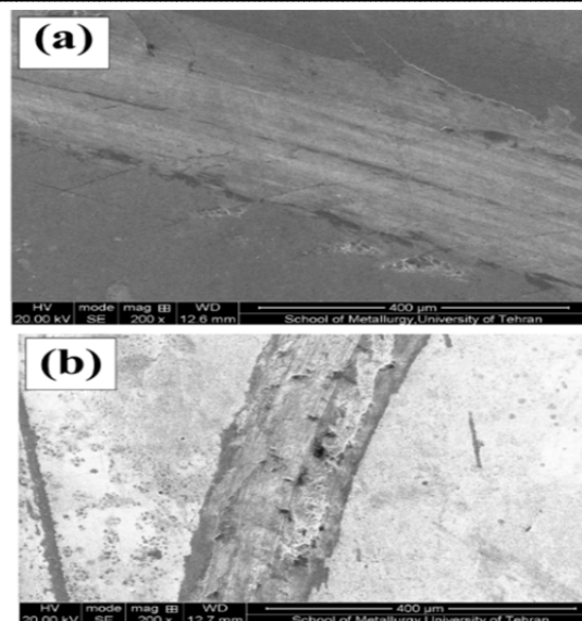
شکل ۷ تصویر SEM سطح سایش پوشش‌های گرا دیانی نیکل-فسفر و نیکل-فسفر-آلومینا بعد از عملیات حرارتی: (a) نیکل-فسفر، (b) نیکل-فسفر-آلومینا بعد از عملیات حرارتی
