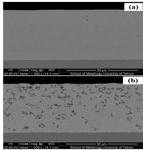
شکل ۳) سطح مقطع پوشش گرادینانی نیکل-فسفر و نیکل-آلومینا: (a) نیکل-فسفر، (b) نیکل-فسفر-آلومینا
