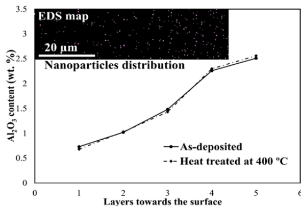
نمودار ۲) مقدار نانوذرات آلومینای موجود در پوشش گرادینانی نیکل-فسفر-آلومینا، قبل و بعد از عملیات حرارتی همراه با نقشه EDS
