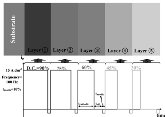
شکل ۲) طرح کلی ایجاد پوشش‌های گرادانی به روش پالس معکوس
