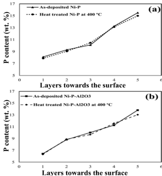
نمودار ۱) مقدار فسفر موجود در پوشش‌های گرادینانی Ni-P و نیکل-فسفر-آلومینا، قبل و بعد از عملیات حرارتی: (a) نیکل-فسفر، (b) نیکل-فسفر-آلومینا
