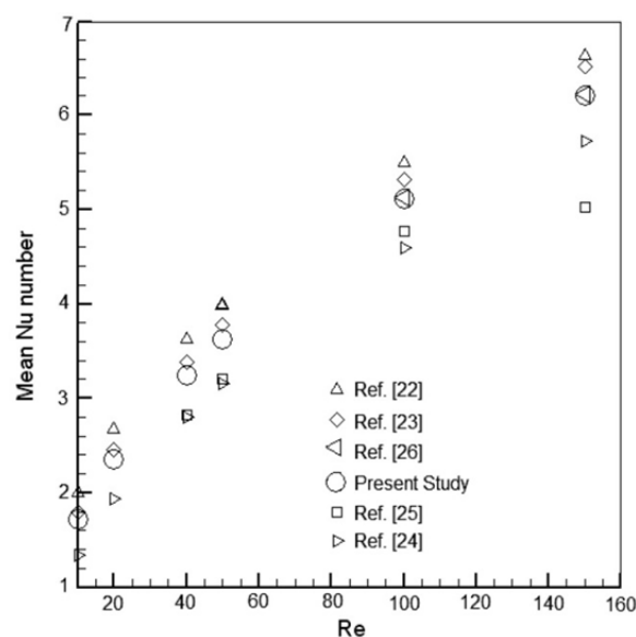
Fig. 16 Comparison of mean Nusselt number around a circular cylinder شکل 16 مقایسه عدد ناسلت میانگین حول استوانه
