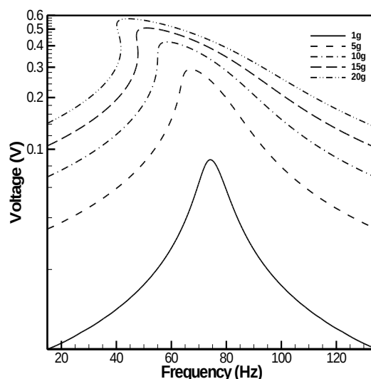
Fig. 7 Voltage, L=50\text{mm} , c=10
