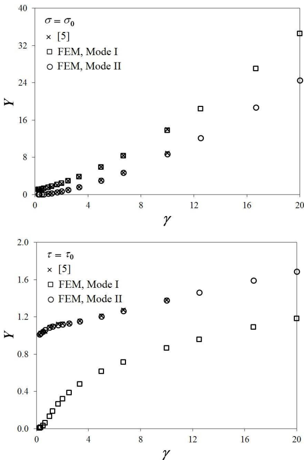
Fig. 7 Comparison of obtained geometry correction factors for subsurface crack by FEM and Ref. [5] under uniform tension and shear شکل 7 مقایسه ضرایب شکل به دست آمده از حل اجزای محدود با مقادیر مرجع [5] برای ترک زیرسطحی تحت کشش و برش یکنواخت
