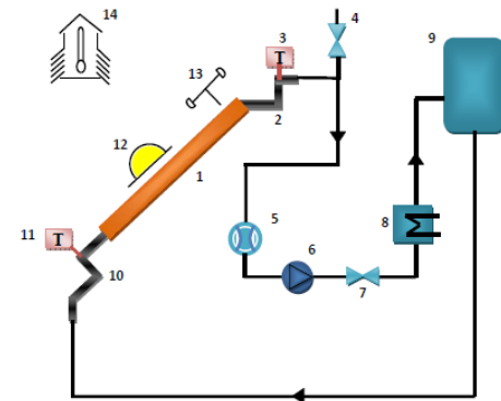
1) Collector 2) Insulated Pipe 3) Temperature Sensor 4) Air Vent 5) Flowmeter 6) Pump 7) Control Valve 8) Circulating Bath 9) Expansion Tank 10) Insulated Pipe 11) Temperature Sensor 12) Pyranometer 13) Anemometer 14) Ambient Air Temperature Sensor
