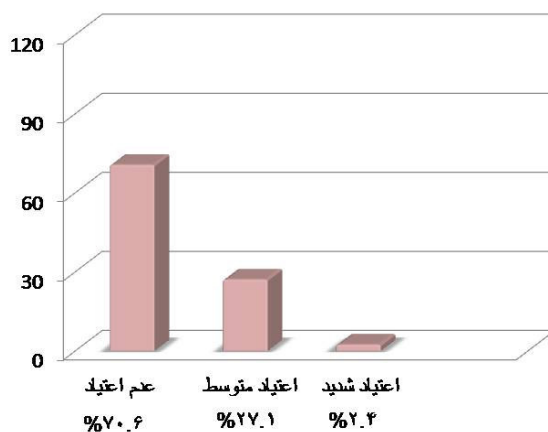
شکل ۱ تحلیل داده‌ها
